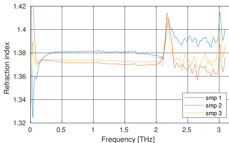
Rysunek 21. Współczynnik załamania dla badanych próbek histydyny prześwietlanych wiązką laboratoryjnego spektrometru w paśmie THz.
