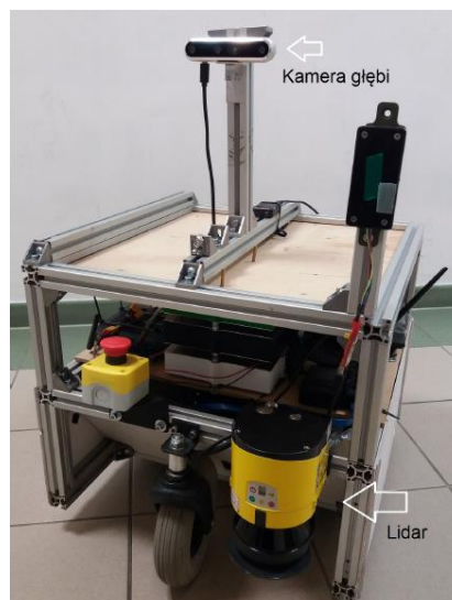
Rys. 7. Prototyp autonomicznego robota mobilnego
