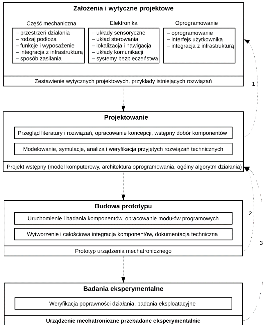
Rys. 1. Proces projektowania robotów mobilnych w ujęciu mechatronicznym
