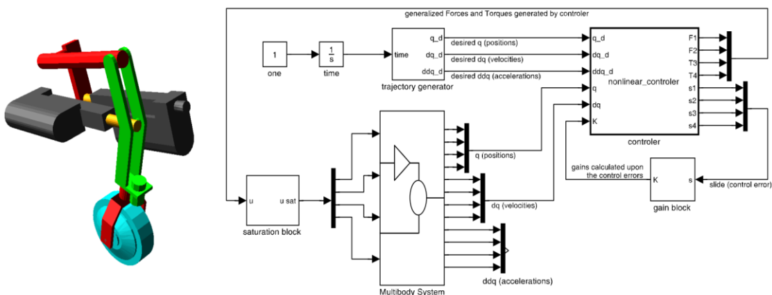
Rys. 2. Widok modelu dynamiki oraz struktura układu sterowania
